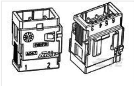
TE 产品编号282994-2 TAB CONN.NEW GEN.F.TRUCK
