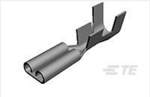
TE 产品编号41771-1 250 FASTON REC 22-18 AWG BR
