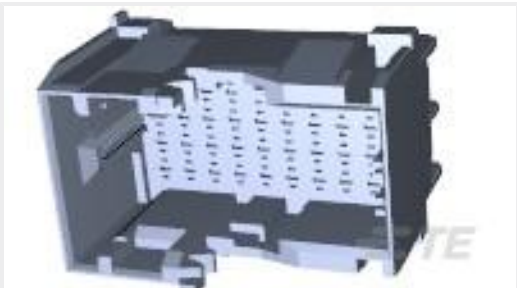
TE 产品编号172076-2 PL MKII 250 REC HSG 1P NYLON BLACK
