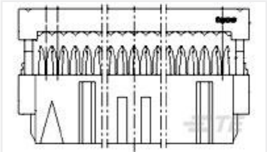
TE 产品编号5-215882-0 50 WAY BLACK MK II RECEPT
