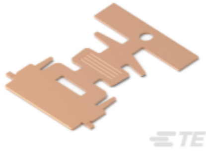
TE 产品编号1-1600961-7 CONT 12-16 AWG PWR, MFBL PLATE
