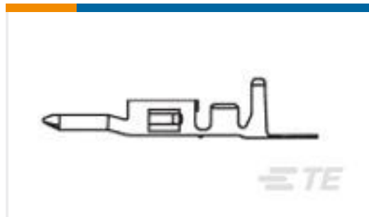
TE 产品编号794957-2 VAL-U-LOK PIN BR AU 22-26AWG
