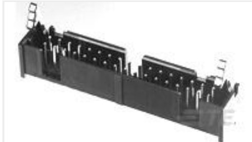
TE 产品编号3-1761606-5 IDC LOW PRO HDR 50P VERT LA
