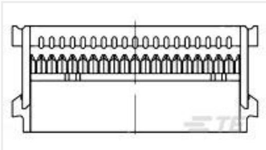
TE 产品编号2-1658526-9 609-1630LF=FSKT IDC S 16 30AU
