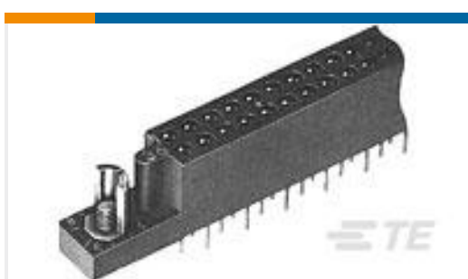
TE 产品编号531129-3 2 ROW BOX RECP 20 POS STAG
