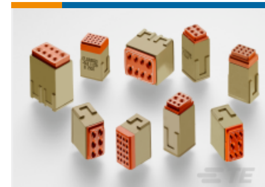
TE 产品编号CTJ122E01C-513 MODULE ASSY
