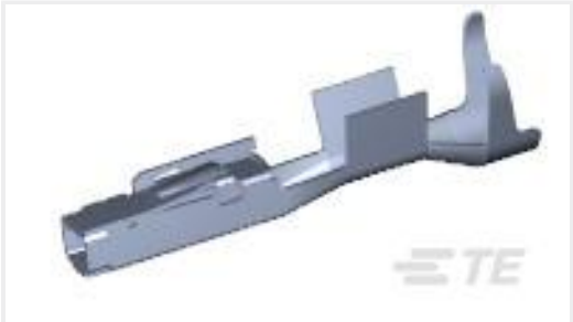
TE 产品编号7-1452671-1 MCON 1.2 LL REC SWS SN
