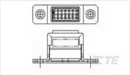
TE 产品编号592840-1 TJ F/B 21E34-699
