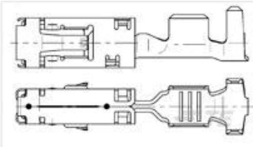
TE 产品编号967543-1 SENSOR FLA-KONT 2,8
