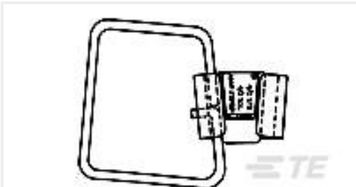
TE 产品编号602115 AMPACT STIRRUP ASSY
