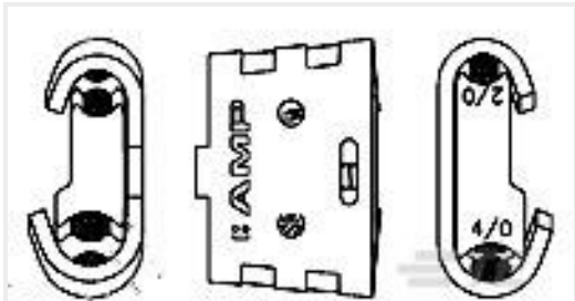
TE 产品编号83631-7 MINI WEDGE, 200AMP, 2/0-#2
