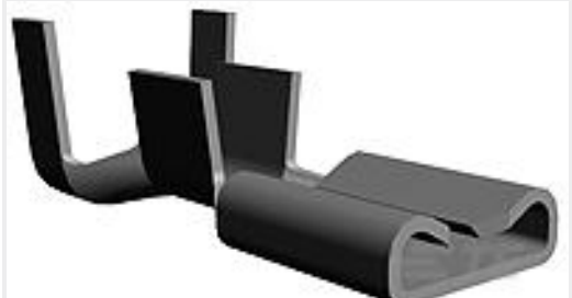
TE 产品编号63347-1 187 FASTON REC 22-18 AWG BR
