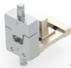
TE 产品编号2378425-1 DIE SET IPT-180 T 95MM2
