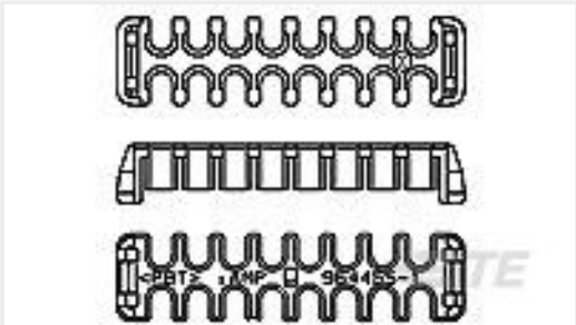
TE 产品编号964455-1 KONTAKTSICHERUNG16P
