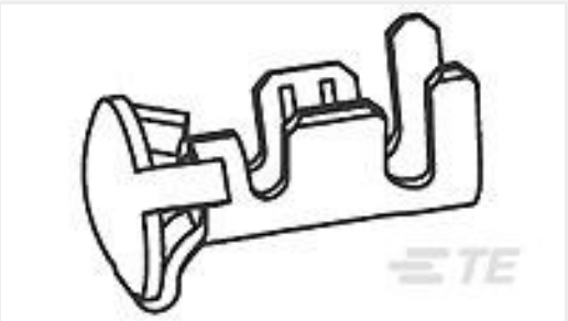
TE 产品编号61165-1 BUTTON CONTACT 20-16 AWG BR
