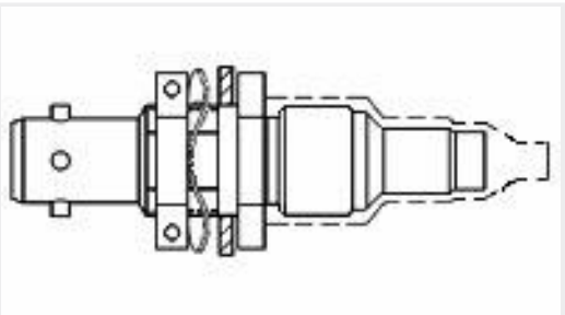
TE 产品编号 042871-000 DK-621-0440-4P
