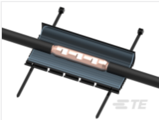
TE 产品编号 C42628-000 GELWRAP-18/4-200(B6)-DE
