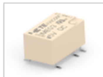
IME03GR=IM RELAY 140mW 5V 2NO
