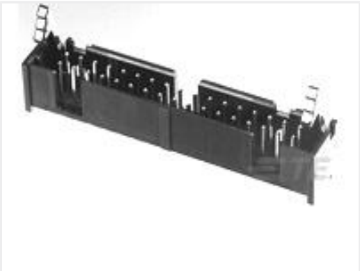
TE 产品编号3-1761606-1 IDC LOW PRO HDR 34P VERT LA
