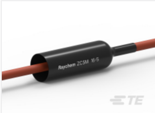
TE 产品编号 342016-000 ZCSM-16/5-1000/U
