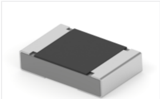
TE 产品编号2176478-6 RA73F 2A 6K65 0.1% 1K RL
