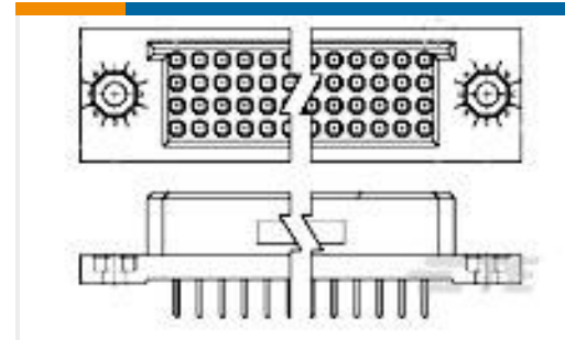
TE 产品编号1-533285-2 BOX II 4 ROW RECP ASSY 300 POS
