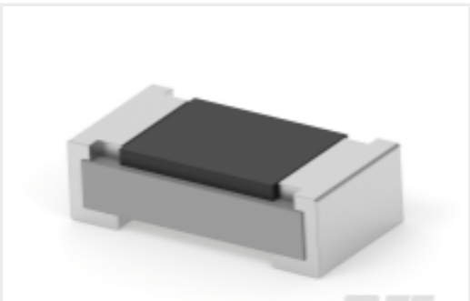
TE 产品编号4-2176090-2 RP 1J 0.166W 1K0 0.1% 25PPM 5K RL
