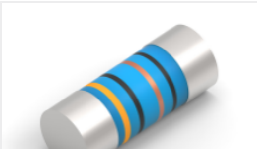
TE 产品编号9-2176314-0 MELF SMA-A 390K 1% 50PPM 0102 0.3 W
