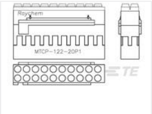
TE 产品编号603431-000 MTCP-122-20P1
