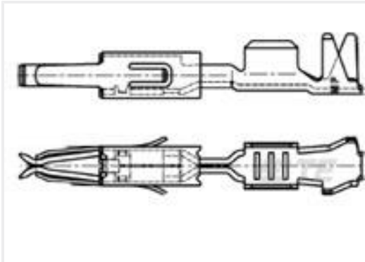
TE 产品编号4-1241732-1 MT3 REC 1.6 Contact SRC Au
