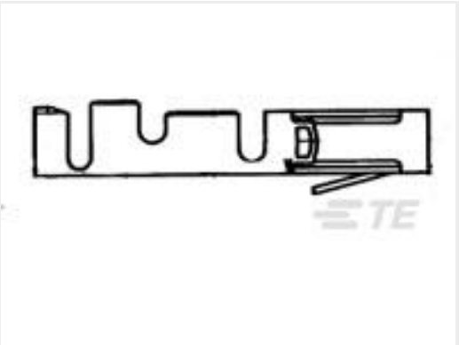
TE 产品编号141098-6 MOD-4 REC.CONTACT
