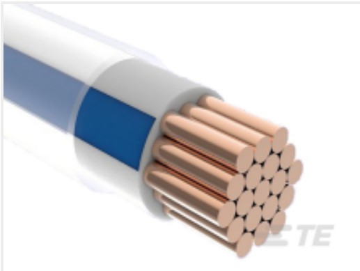
TE 产品编号D798513001 ACW0219-1.00-2(NS)
