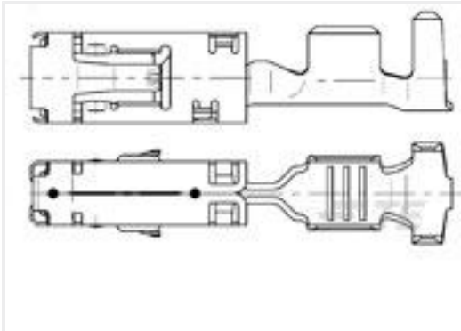
TE 产品编号967542-2 SENS FLA-KONT 2,8
