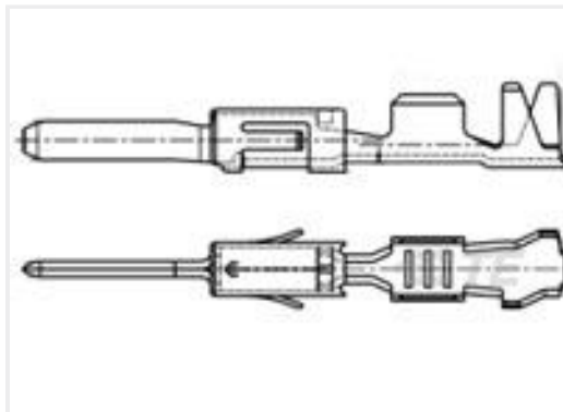
TE 产品编号963904-2 TAB A 1.6x0.6 CONTACT CF SWS Sn
