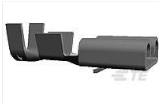
TE 产品编号160860-4 FF 250 REC 0.5-1.0MM2 TPPB
