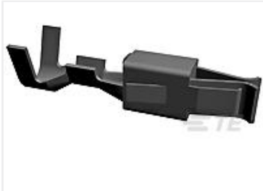
TE 产品编号927766-3 JPT REC 2.8 Contact SWS Sn
