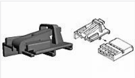
TE 产品编号1418776-1 COVER,MQS,5 POS.
