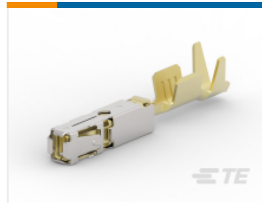
TE 产品编号1534334-3 AMP MCP 1.5K, CONTACT
