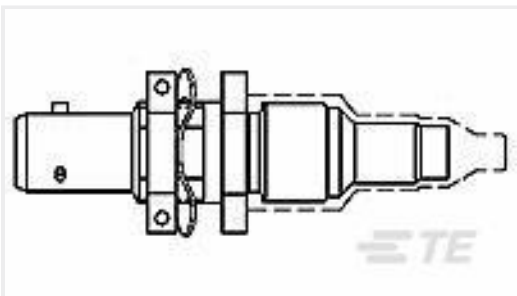
TE 产品编号928733-000 DK-621-0934-1S
