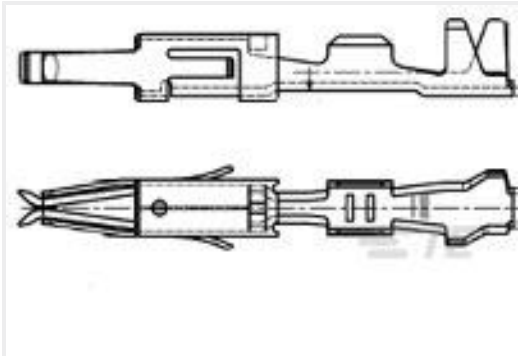
TE 产品编号962876-1 MT2 REC 1.6 Contact SWS Sn
