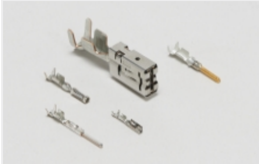
汽车端子(150)
