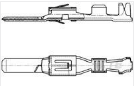
TE 产品编号963814-2 TAB 2,8 SPEC
