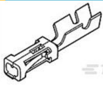
TE 产品编号86016-5 MOD IV RECP LP
