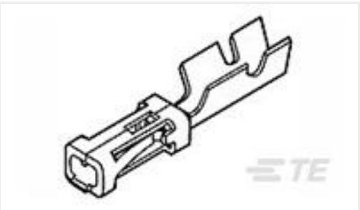
TE 产品编号166310-2 MOD-5 REC.CONTACT
