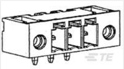
TE 产品编号284539-8 8 POS TERMI-BLOK 900 W.S.F. 3,
