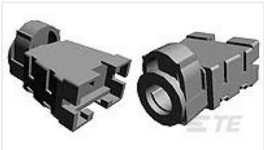
TE 产品编号794370-1 08P MINI UMNL STR RELIEF HNGD
