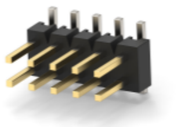
TE 产品编号 1-2271743-0 AMPMPDU PIN HDR 2.54 PITCH 2ROW SMT
