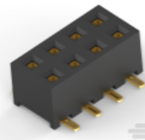
TE 产品编号 2271597-8 AMPMODU, REC HDR, DR, 2.0 PITCH, SMT, 8P
