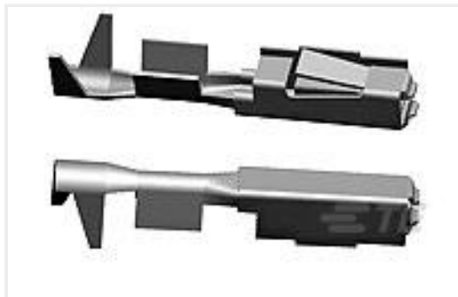
TE 产品编号1355717-1 MQS0,63 Sn rec LL unseal. 0,08-0,22
