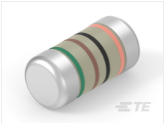
TE 产品编号 9-2176655-8 MELF SMA-Q R261 1% 50PPM 0204 0.4 W
