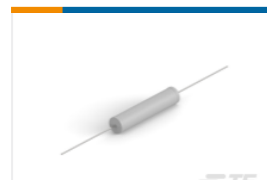
TE 产品编号9-2176415-0 8W STD M/OX 5% 150K
