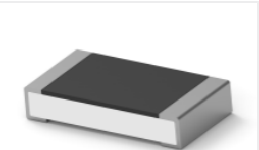
TE 产品编号1-2176387-4 RQ 1206 182K 0.1% 10PPM 1K RL
