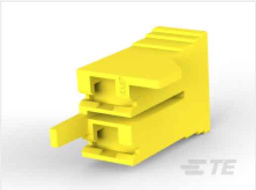
TE 产品编号1-1969232-3 250 FASTON HSG.,REC.,2 POS, YELLOW
